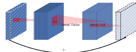
MBConv
